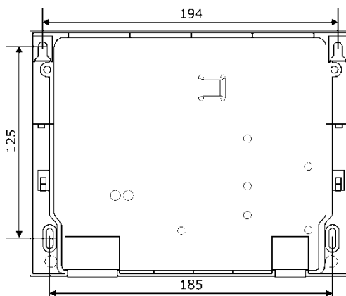
Рис. 4.1 – Схема крепления корпуса ТВ7
