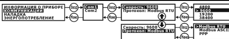
Рис. 3.10 – Настройка Com-портов
