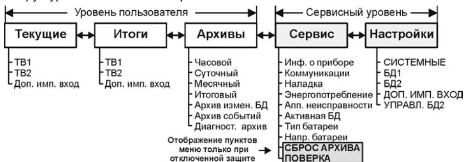
Рис. 2.1 – Структура меню тепловычислителя
