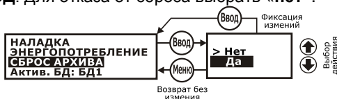
Рис. 3.12 – Сброс архива
