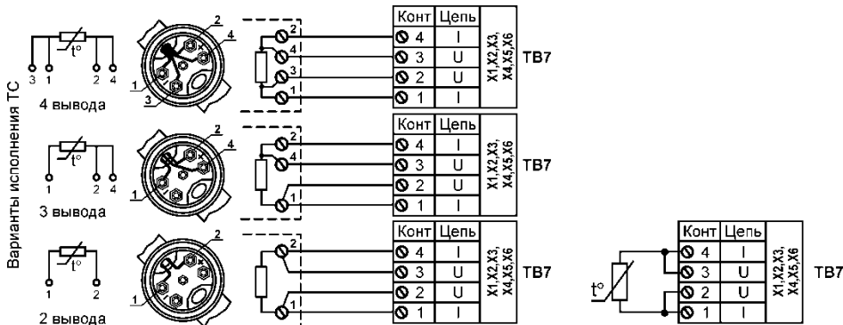
а) Подключение ТС по 4-проводной схеме б) Подключение 2-х проводных ТС
